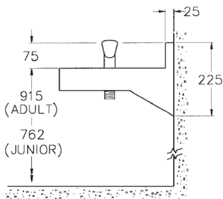
End Elevation
